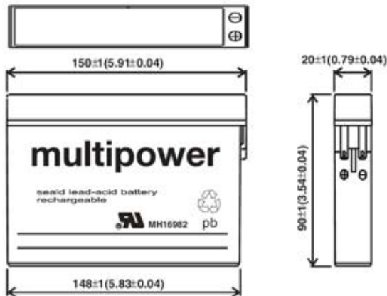
(FASTON TAB NO. 187)
