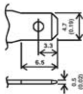
(FASTON TAB NO. 187)
